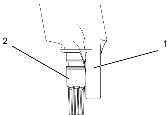
Rysunek 54: Nastawnik odbicia Suntour (2) na widełcu (1)
