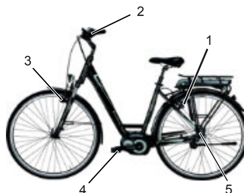
Rysunek 12: Układ hamulcowy roweru typu Pedelec z hamulcem nożnym, przykład
