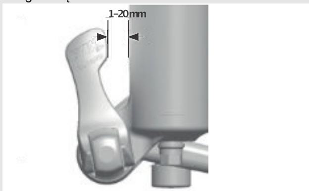
Rysunek 37: Odległość pomiędzy dźwignią a golenią widelca
